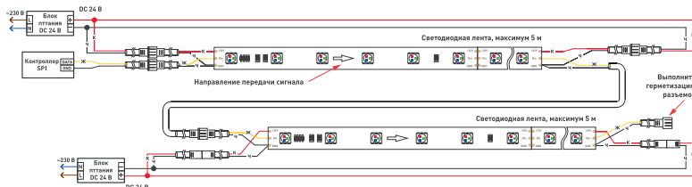
Рис. 3. Схема подключения нескольких светодиодных лент SPI-P-F72 с двух сторон с использованием SPI-контроллера с одним выходным портом и отдельных блоков питания
