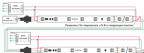
Рис. 1. Схема подключения нескольких светодиодных лент SPI-F72 с двух сторон с использованием SPI-контроллера с одним выходным портом и отдельных блоков питания
